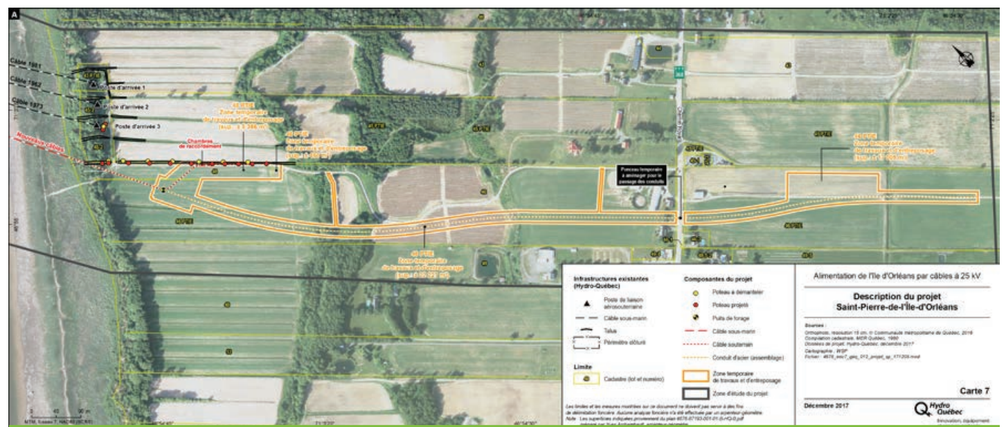
Carte montrant l'emplacement des câbles existants et des futurs conduits.
